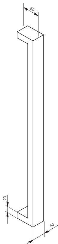
PUXADOR 2100
